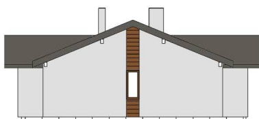
ELEWACJA BOCZNA
