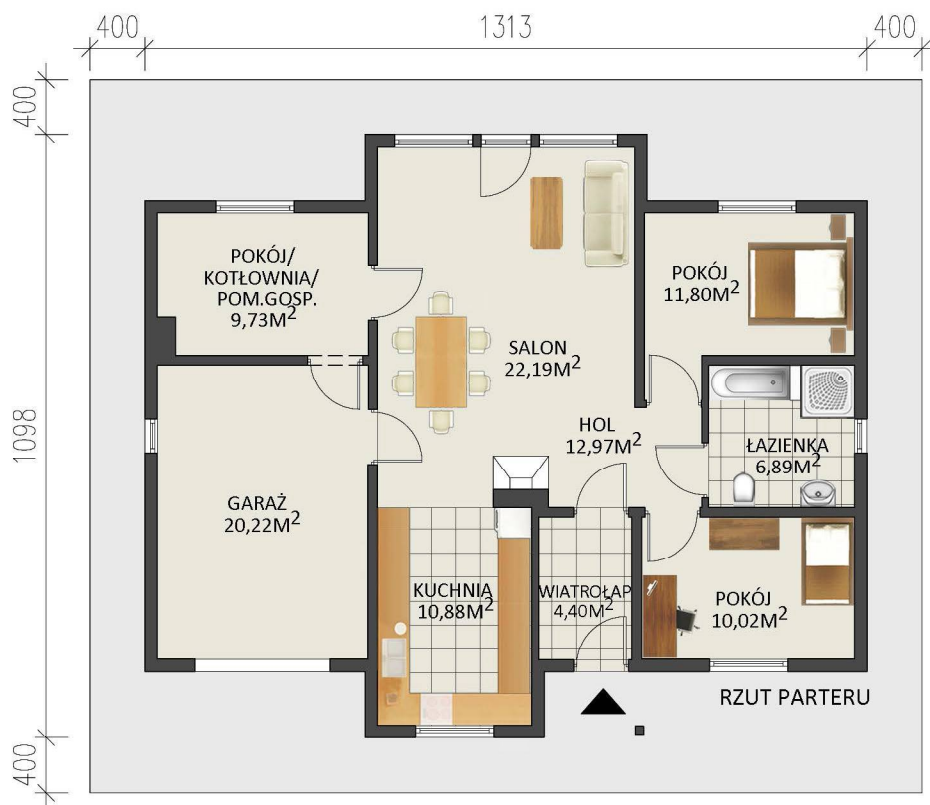
BUNGALOW FIX 89 D MINIMALNE WYMIARY DZIAŁKI 21,13 M X 18,98 M
