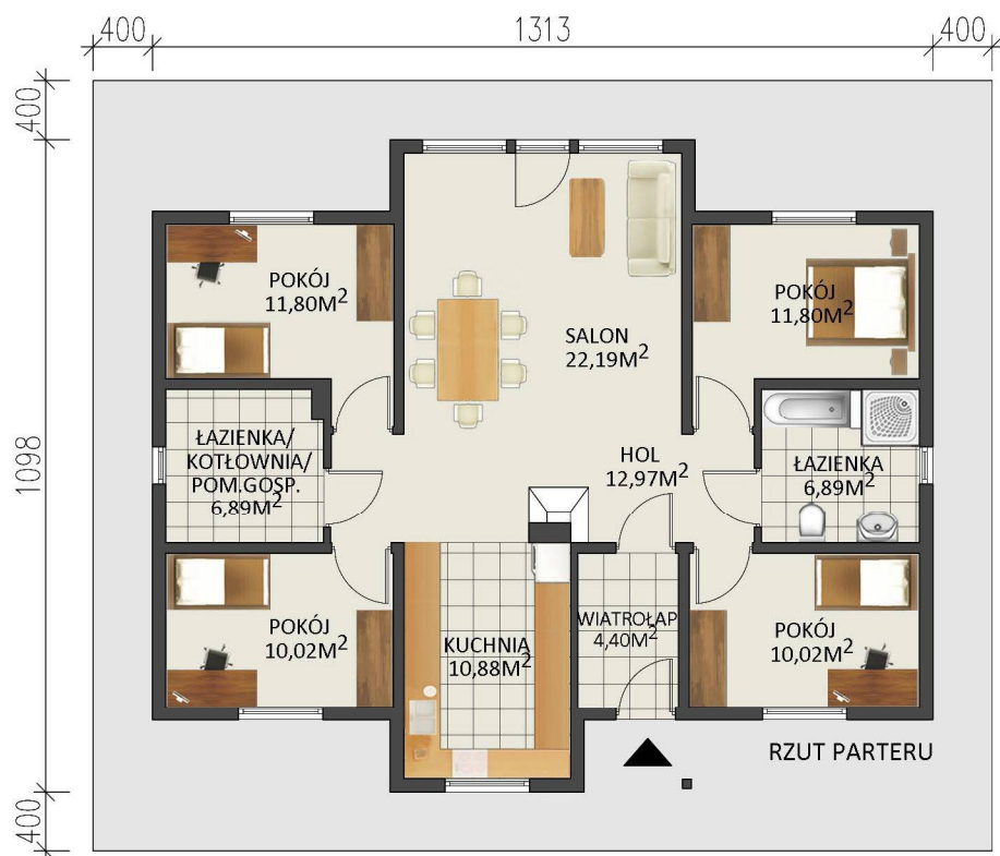
BUNGALOW FIX 107 MINIMALNE WYMIARY DZIAŁKI 21,13 M X 18,98 M
