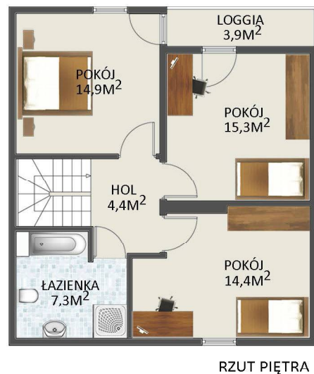
BESKIDY 117 C MINIMALNE WYMIARY DZIAŁKI 22,65 M X 17,25 M
