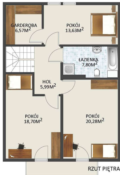
FAMILY 151 B MINIMALNE WYMIARY DZIAŁKI 20,46 M X 18,96 M
