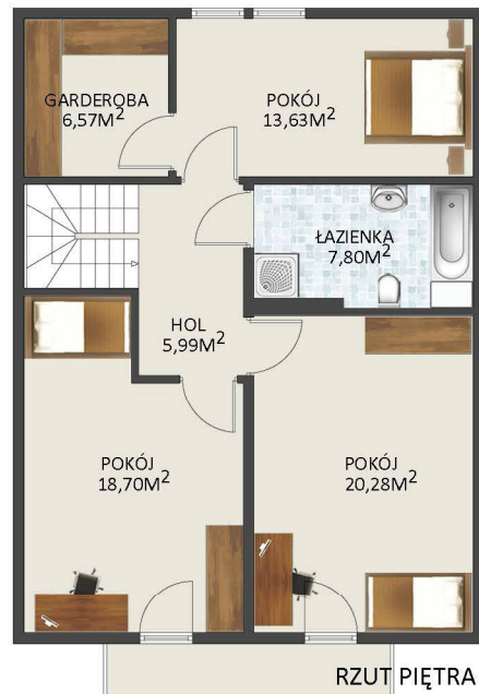
FAMILY 151 C MINIMALNE WYMIARY DZIAŁKI 22,67 M X 18,96 M
