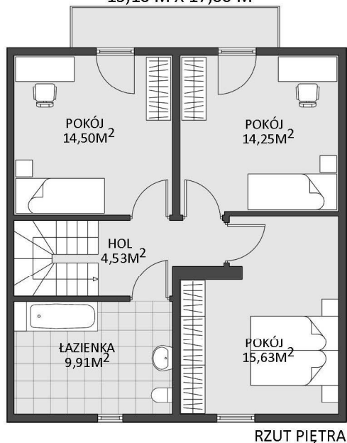
KOMFORT 121 MINIMALNE WYMIARY DZIAŁKI 15,10 M X 17,00 M
