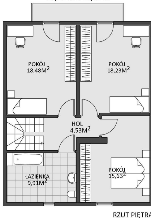
KOMFORT 136 MINIMALNE WYMIARY DZIAŁKI 15,10 M X 18,06 M
