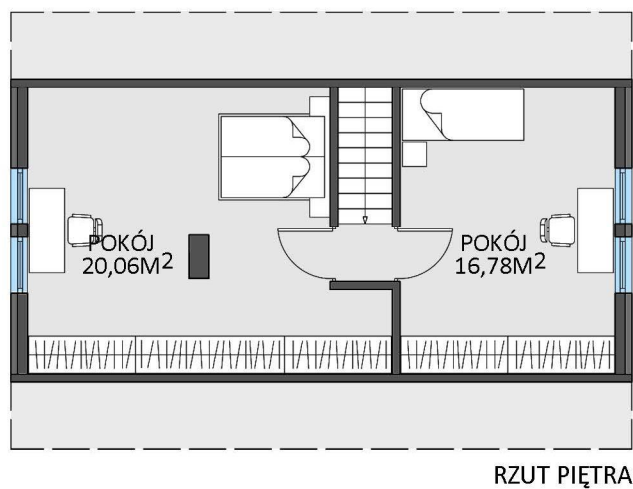
SMART 102 MINIMALNE WYMIARY DZIAŁKI 16,22 M X 15,20 M
