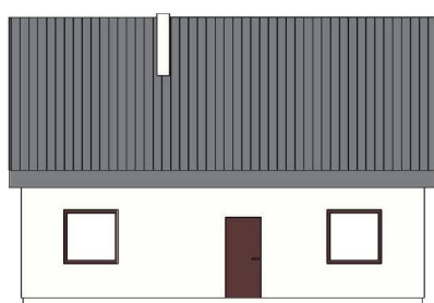
ELEWACJA PRZEDNIA
