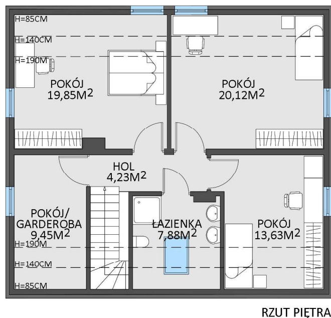
SMART 155 MINIMALNE WYMIARY DZIAŁKI 16,22 M X 17,14 M
