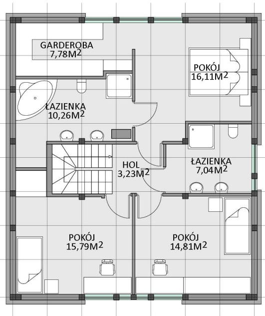
IHAUS 153 SIDE MINIMALNE WYMIARY DZIAŁKI 16,00 M X 18,50 M
