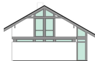
ELEWACJA BOCZNA
