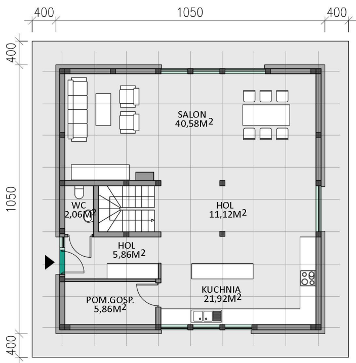
RZUT PARTERU
