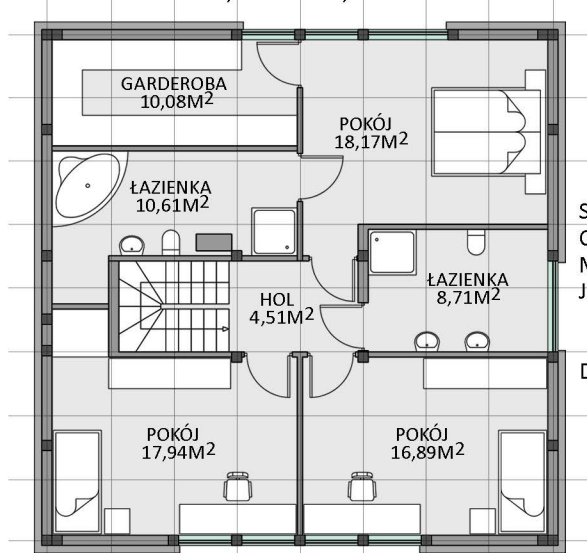
RZUT PIĘTRA
