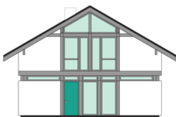
ELEWACJA PRZEDNIA
