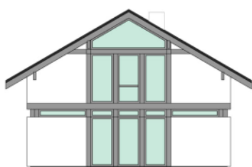
ELEWACJA TYLNA
