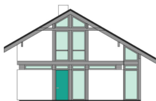
ELEWACJA PRZEDNIA
