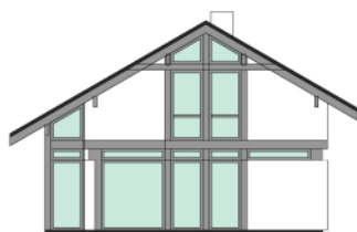
ELEWACJA TYLNA
