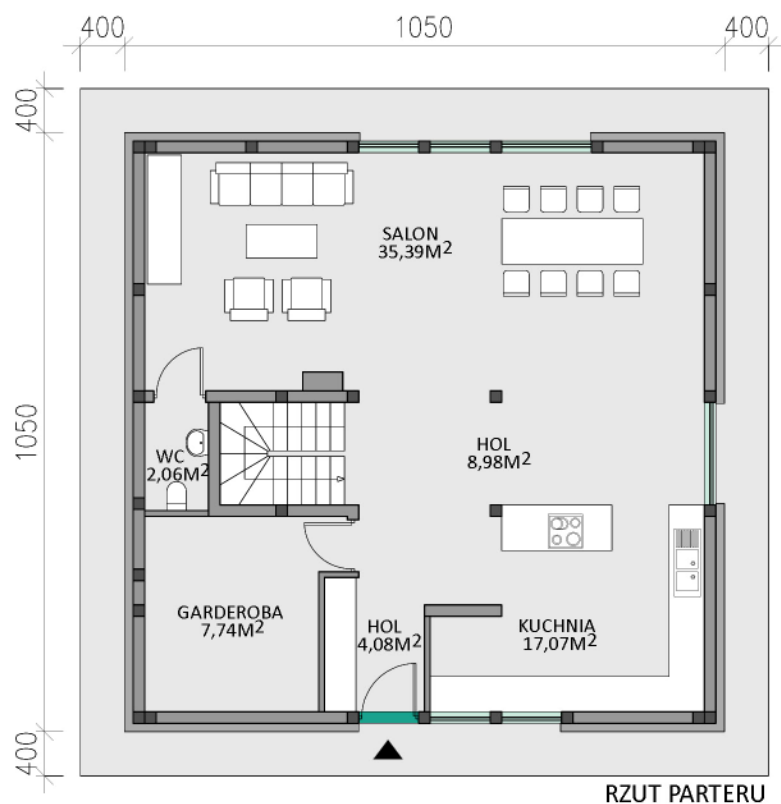
IHAUS 178 FRONT MINIMALNE WYMIARY DZIAŁKI 18,50 M X 18,50 M
