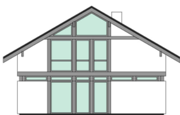
ELEWACJA TYLNA
