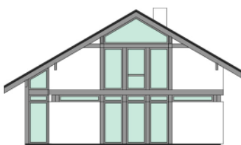
ELEWACJA TYLNA
