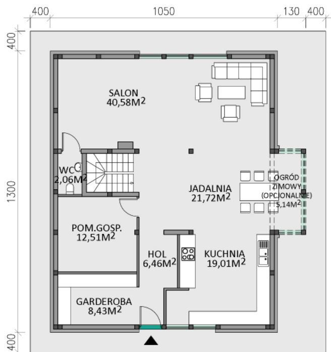
RZUT PARTERU
