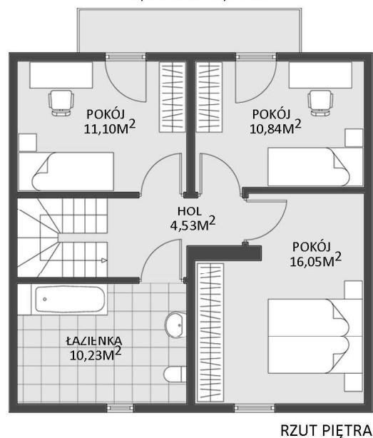
KOMFORT 107D MINIMALNE WYMIARY DZIAŁKI 17,66 M X 16,00 M
