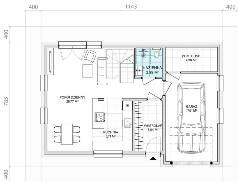
RZUT PARTERU
