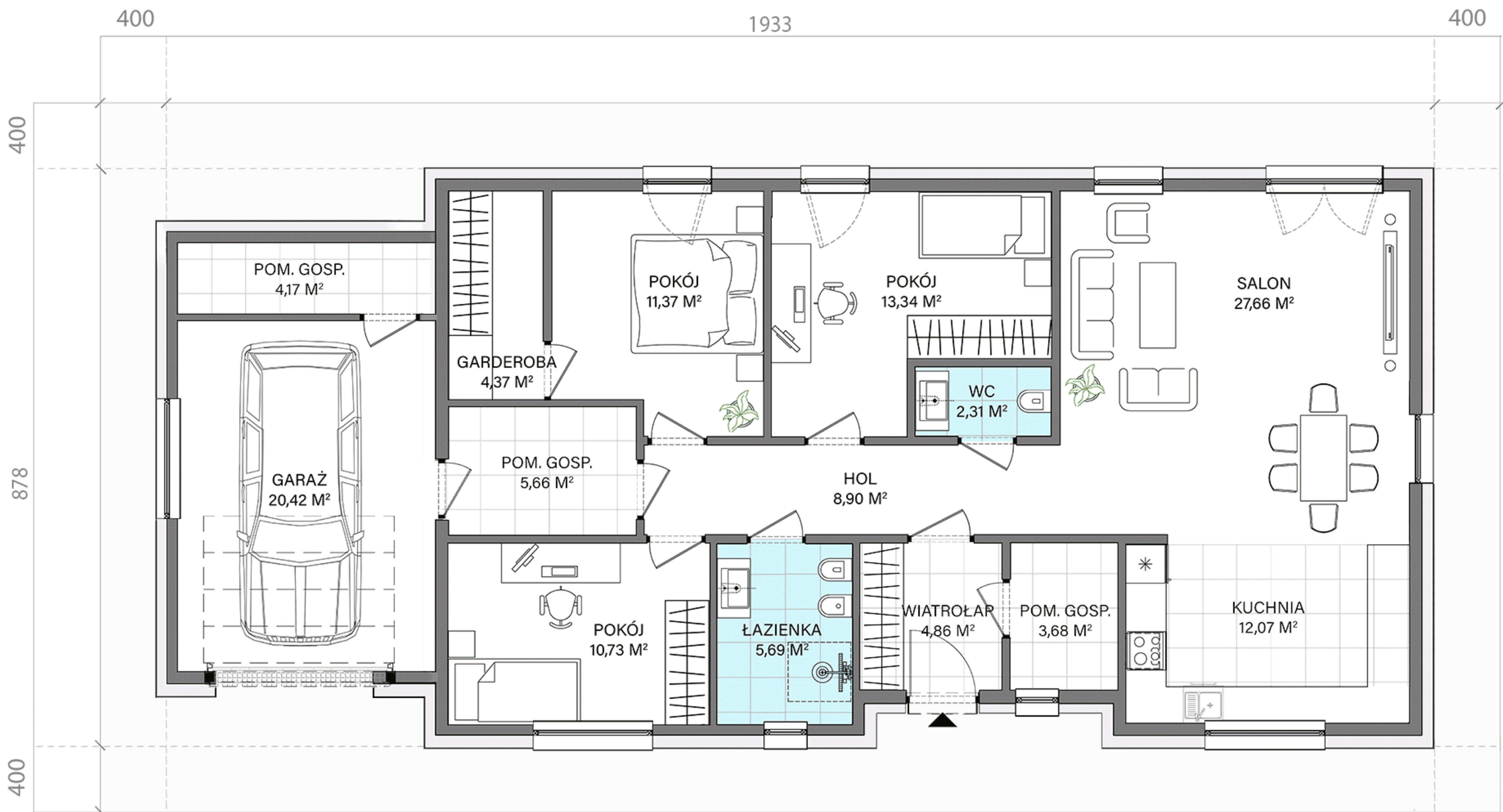
RZUT PARTERU
