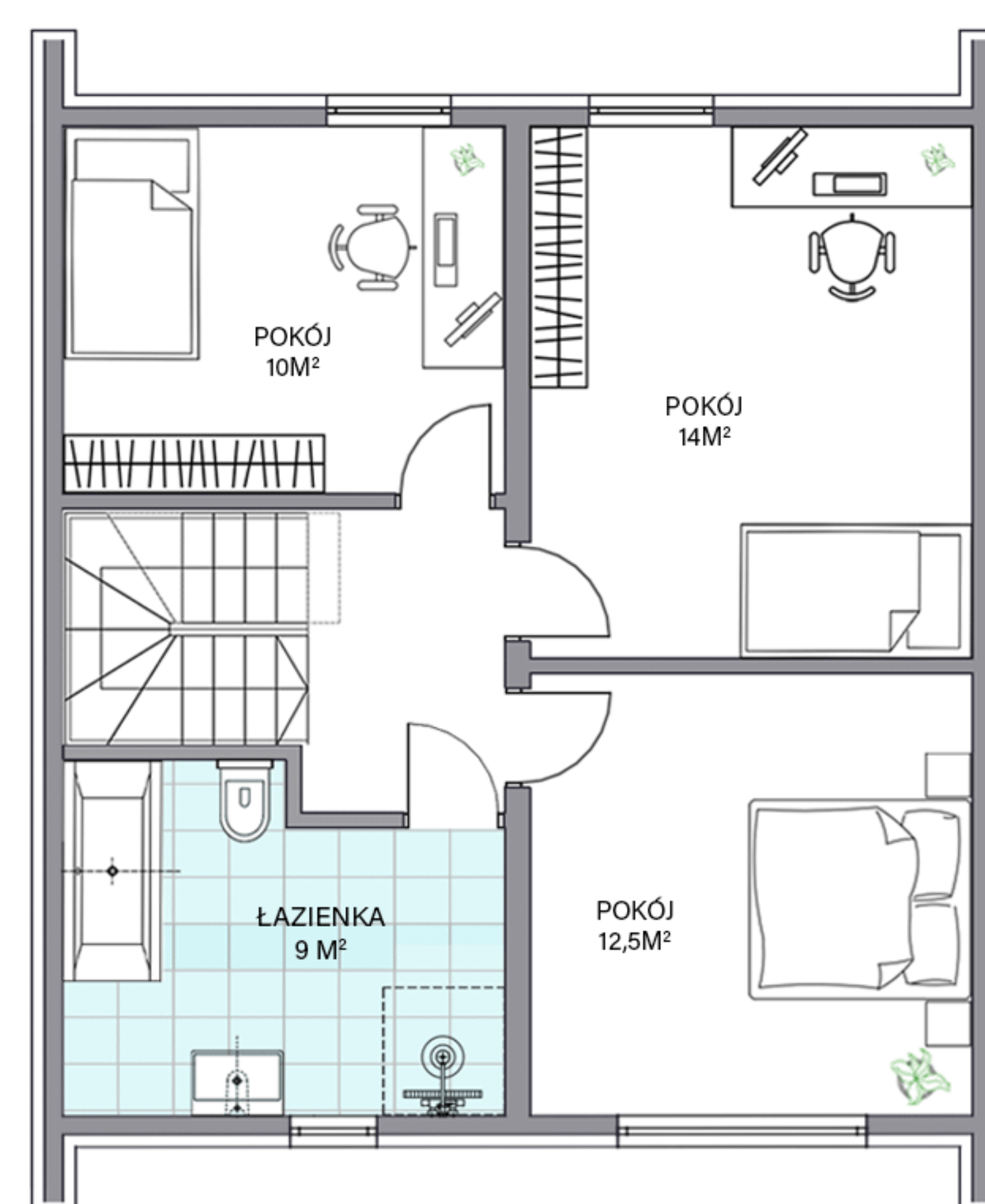
RZUT PIĘTRA
