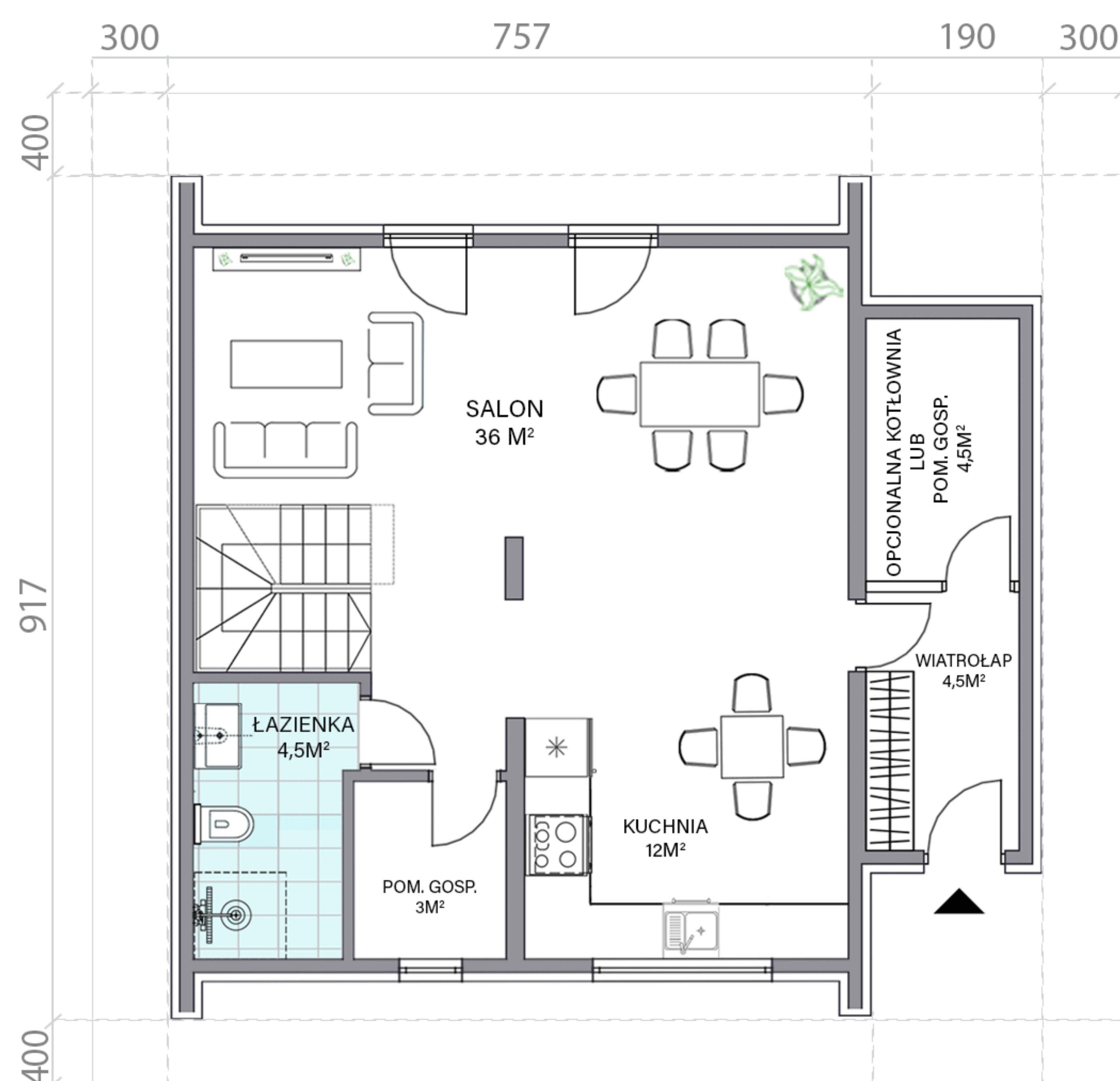
RZUT PARTERU
