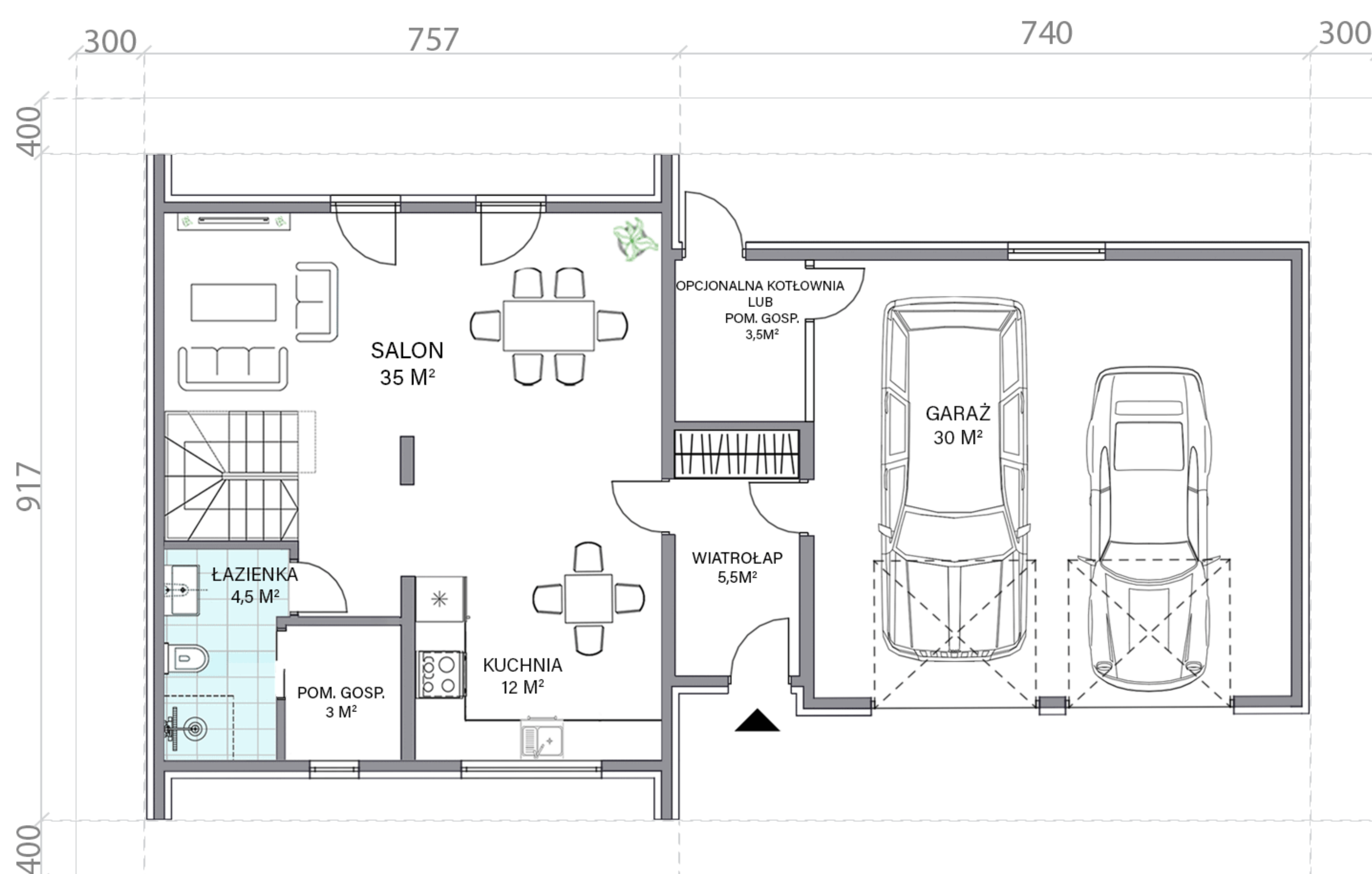
RZUT PARTERU
