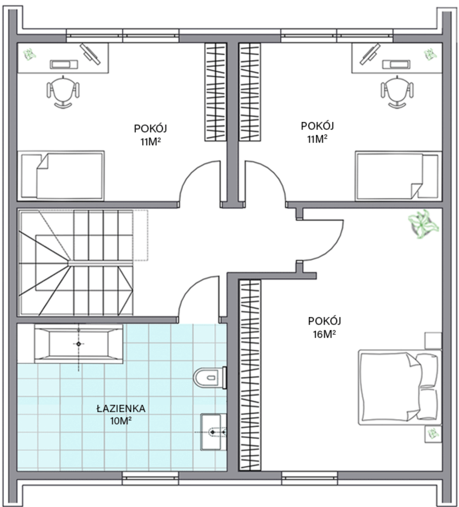
RZUT PIĘTRA
