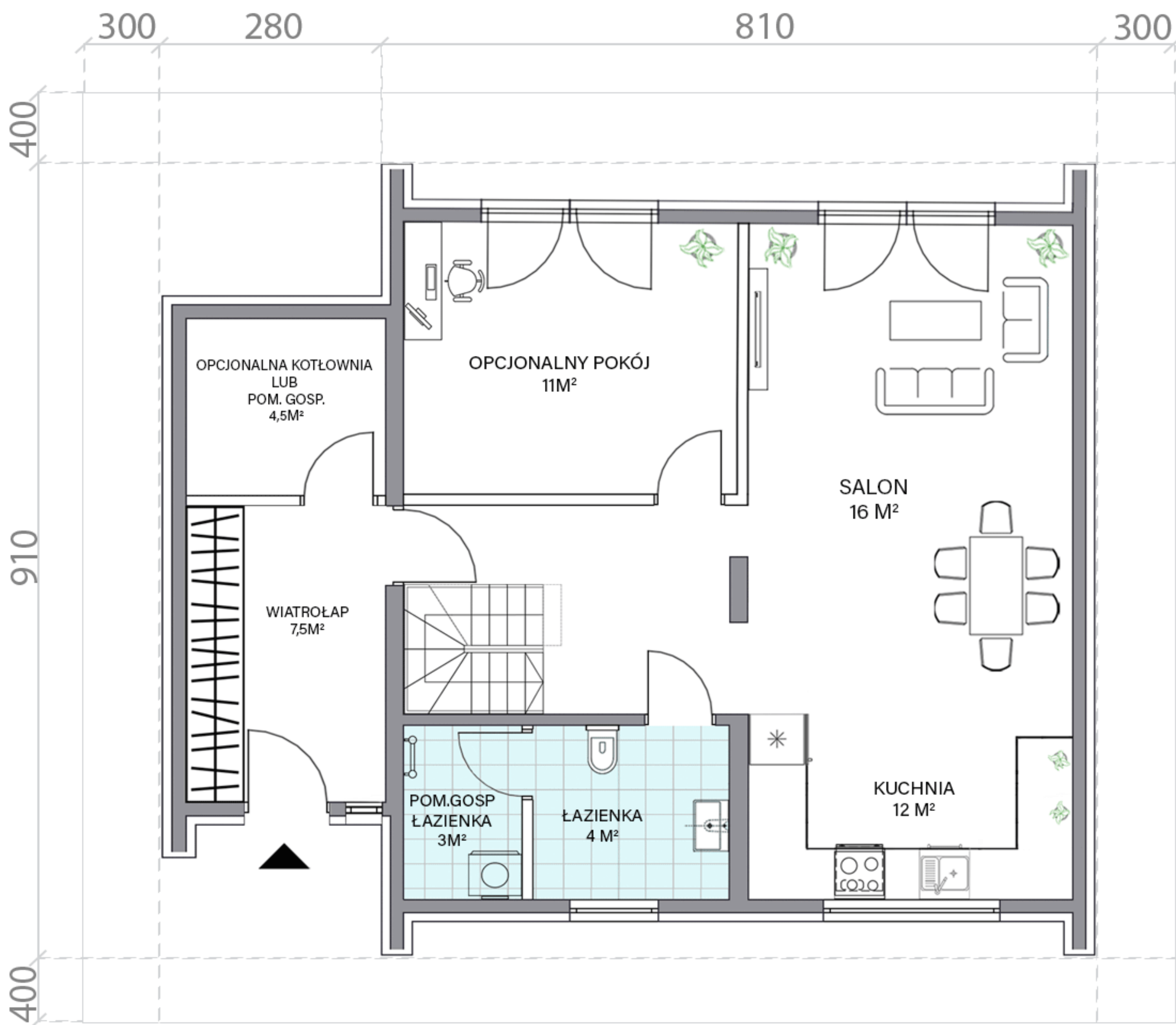
RZUT PARTERU
