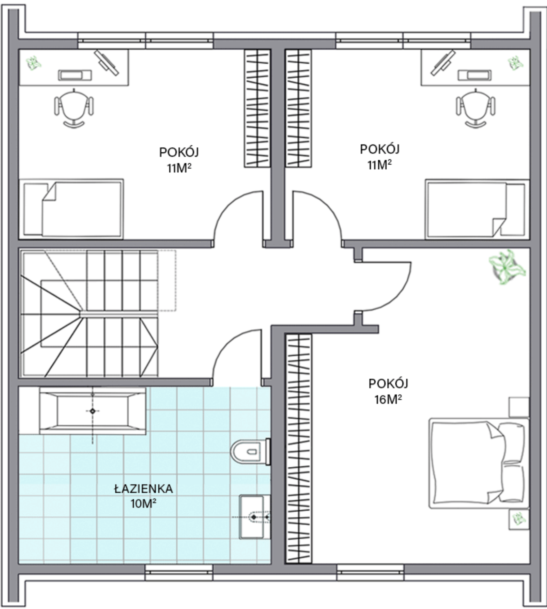
RZUT PIĘTRA
