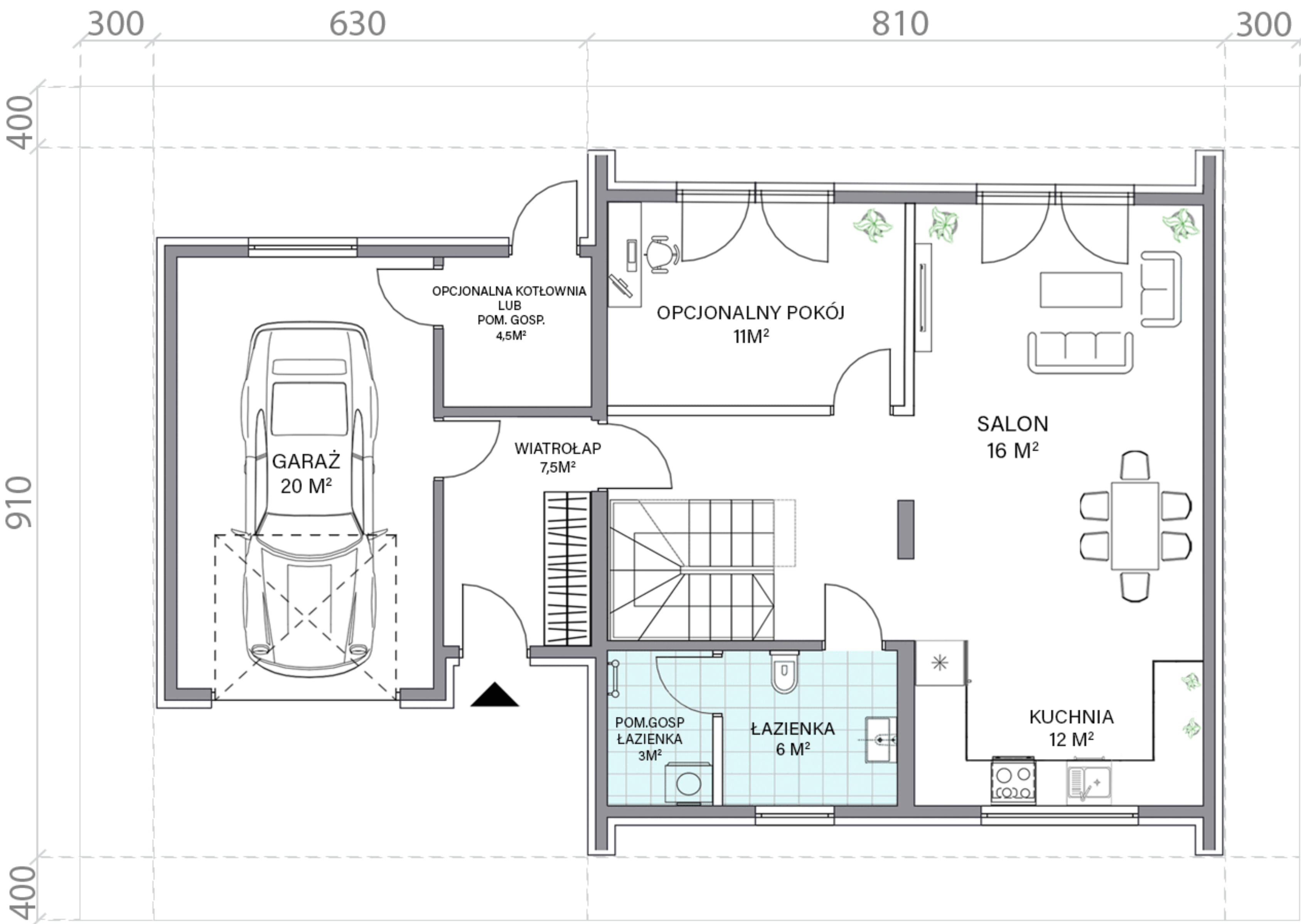
RZUT PARTERU
