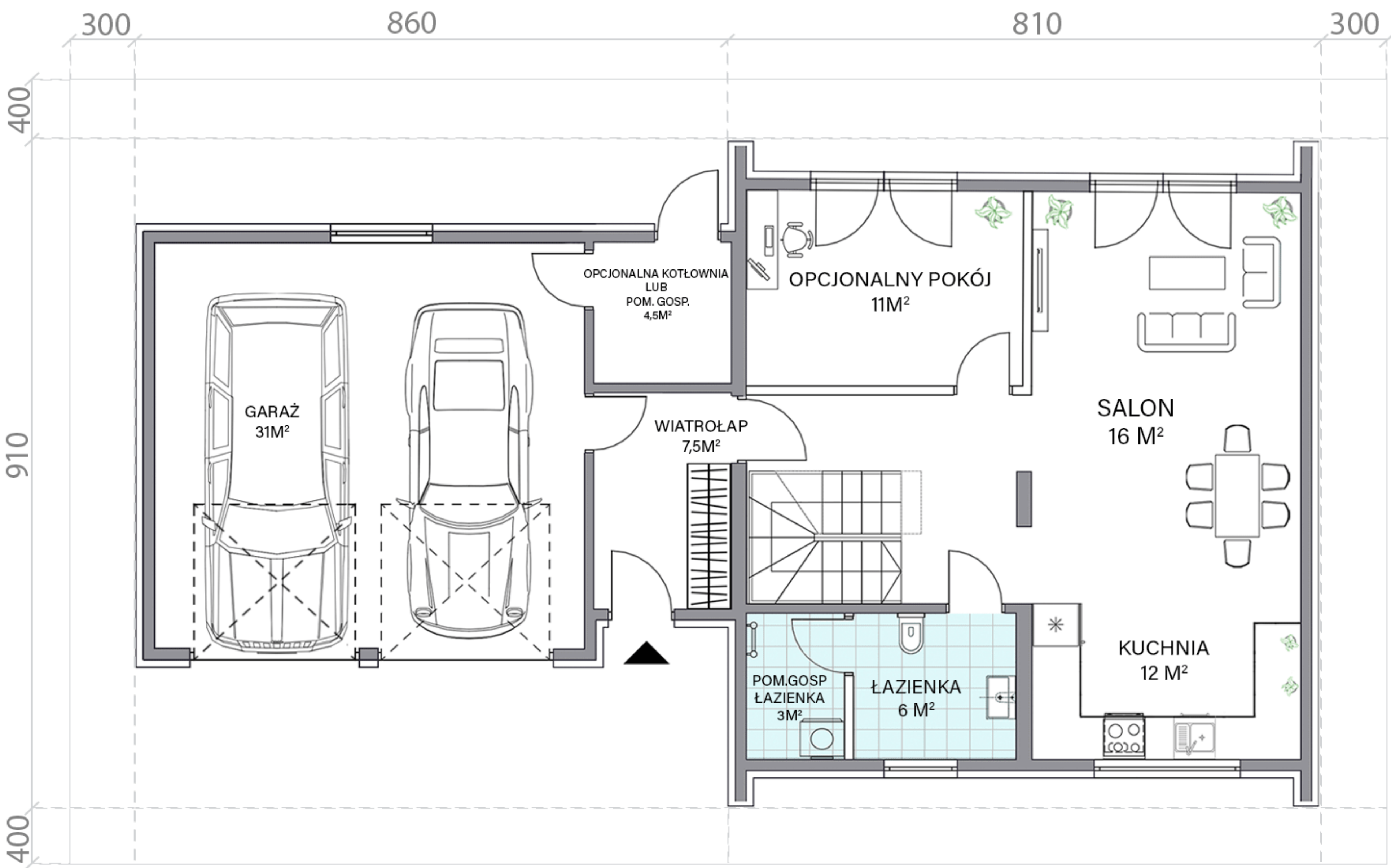
RZUT PARTERU
