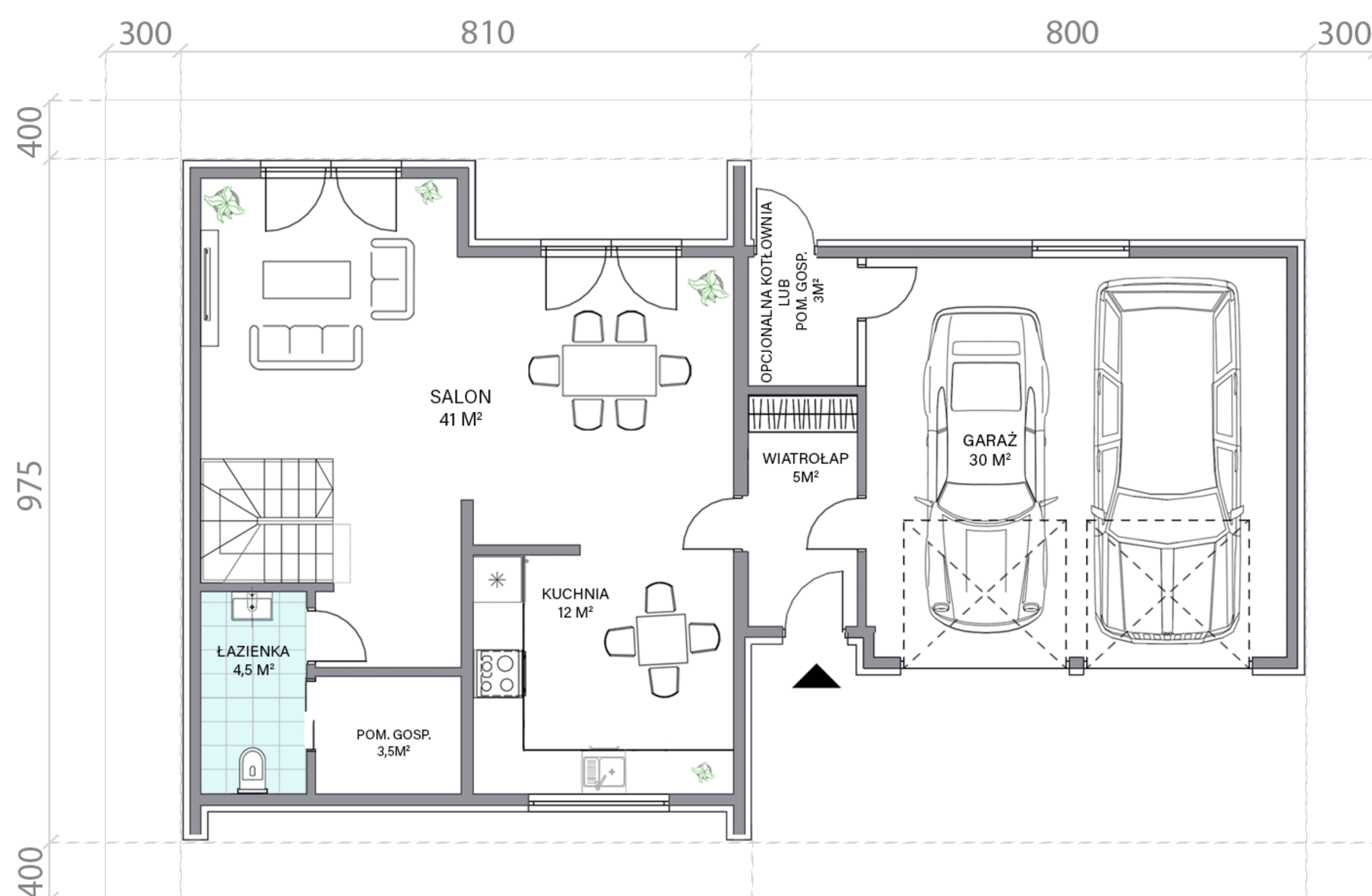
RZUT PARTERU
