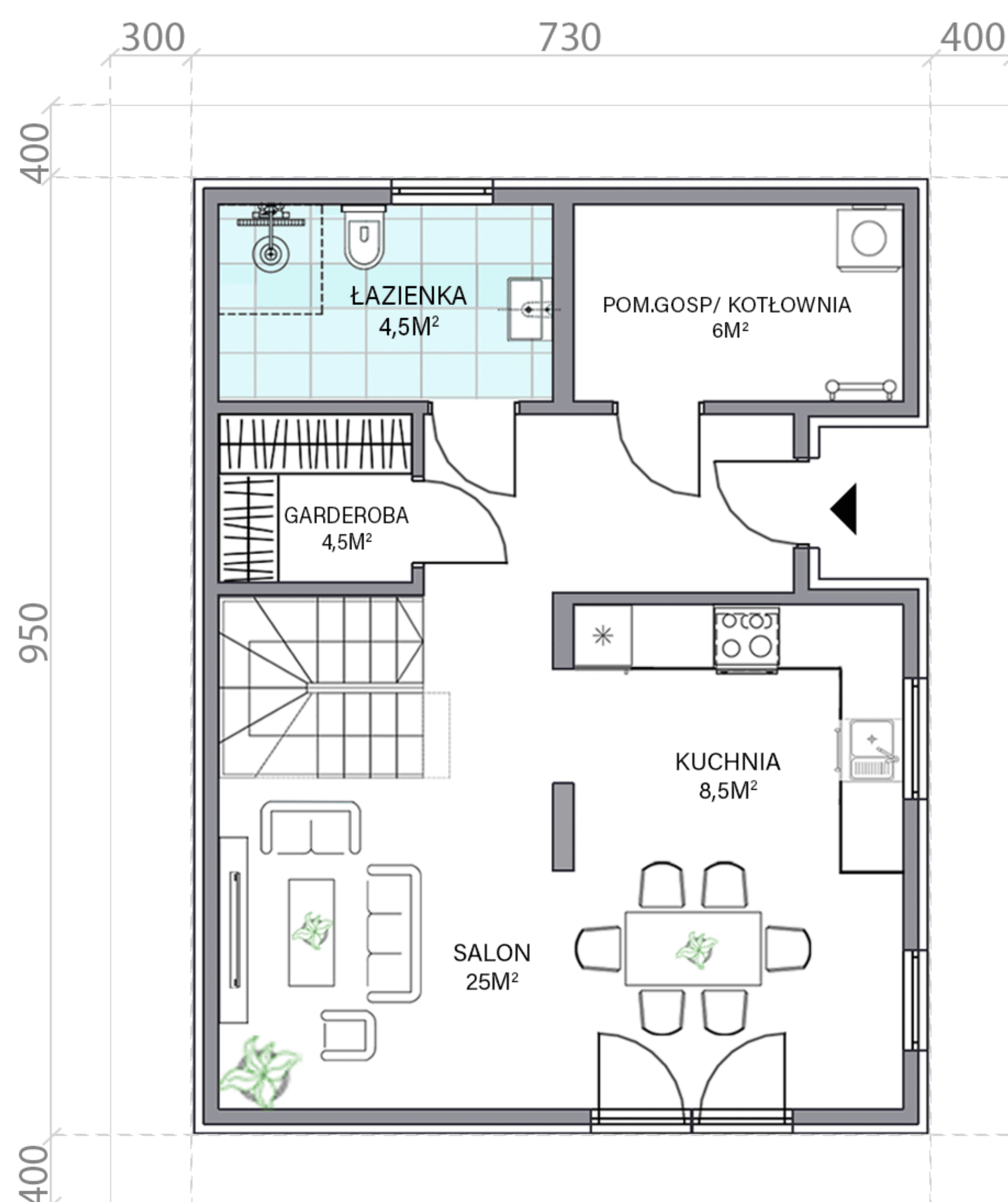
RZUT PARTERU
