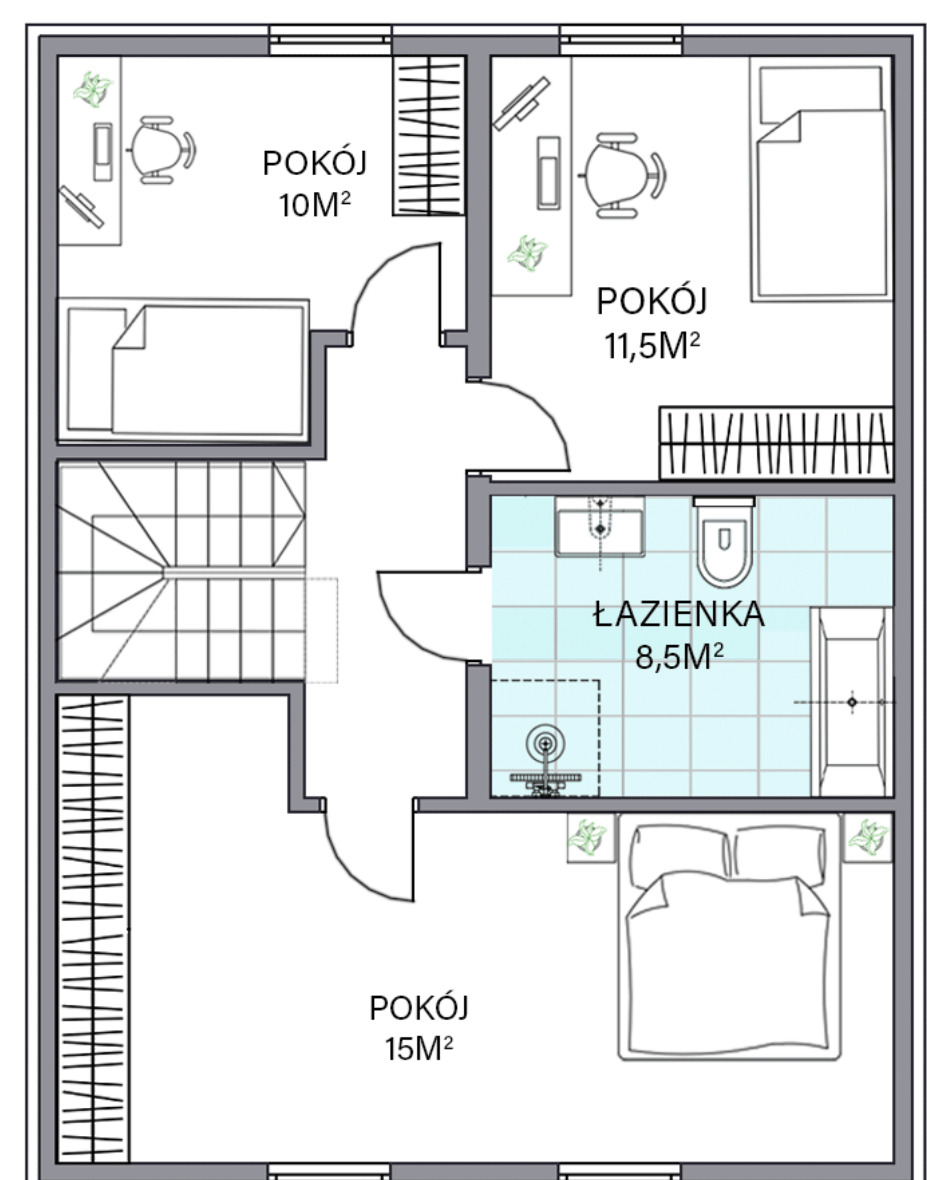
RZUT PIĘTRA
