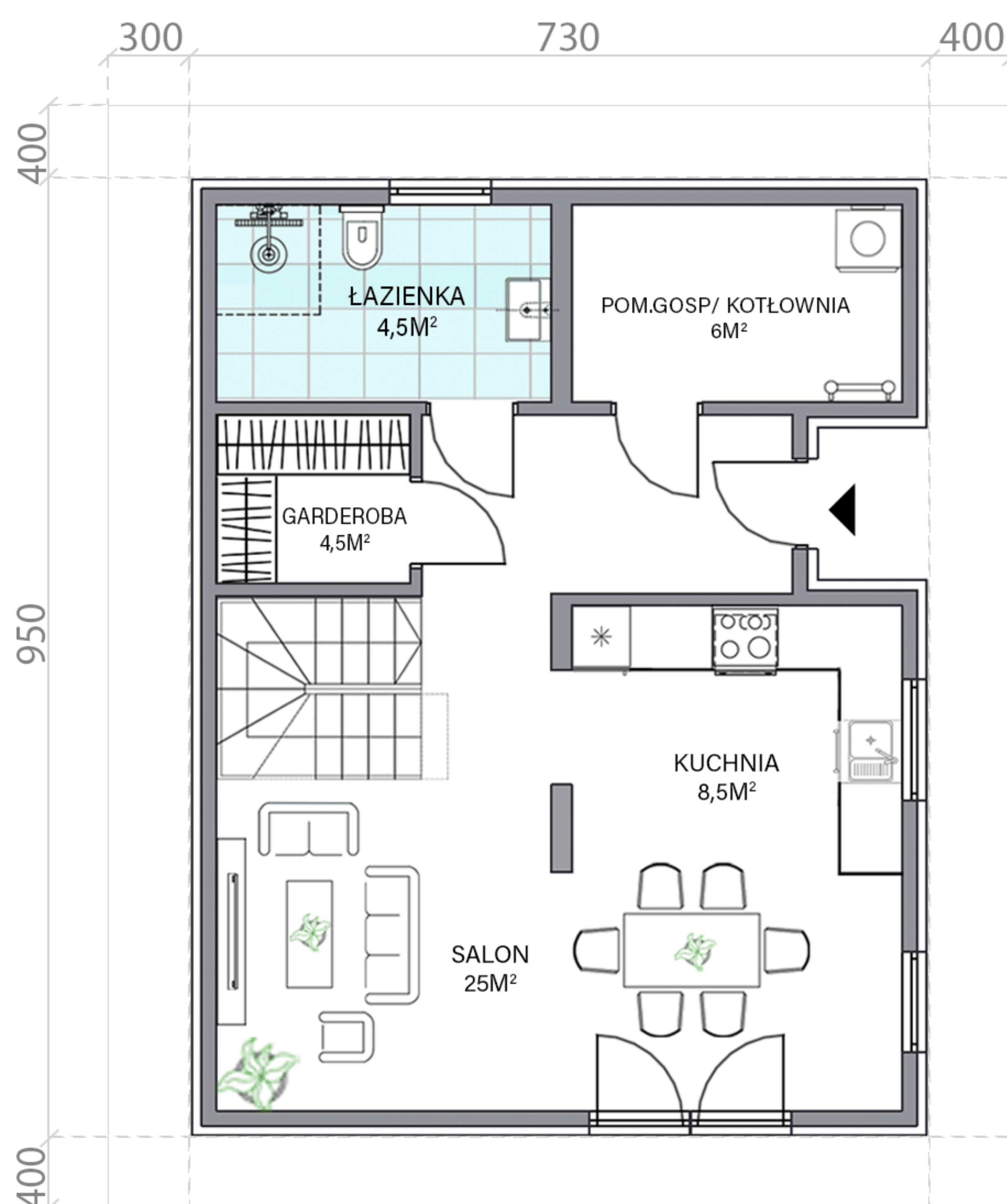
RZUT PARTERU
