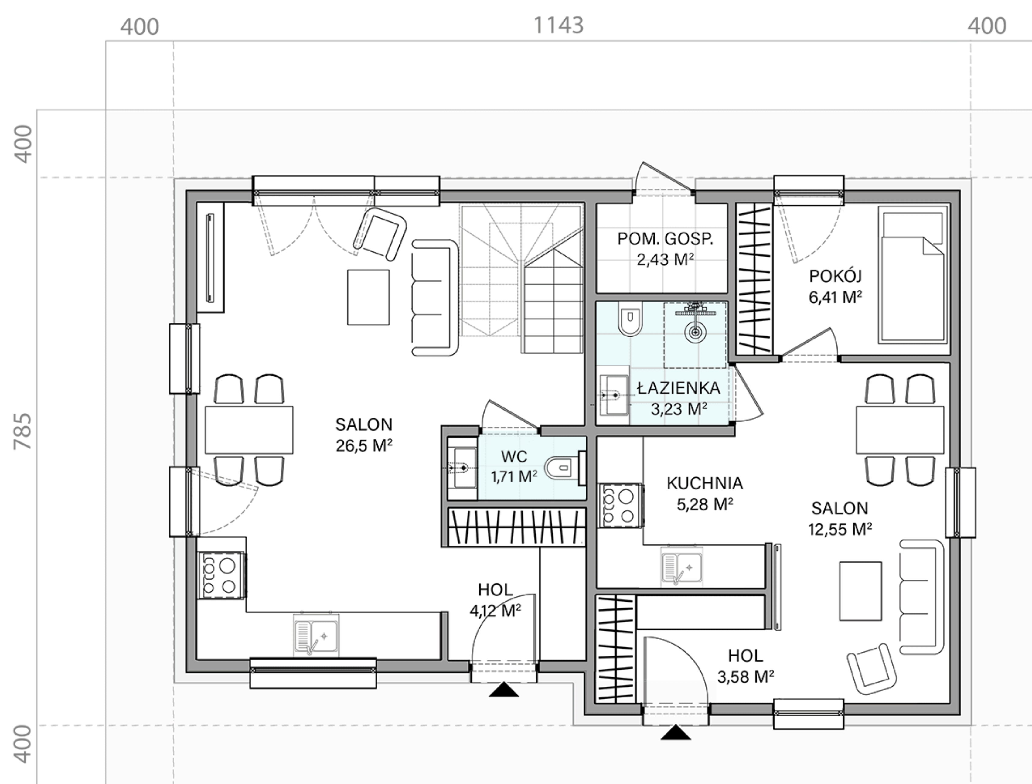
RZUT PARTERU
