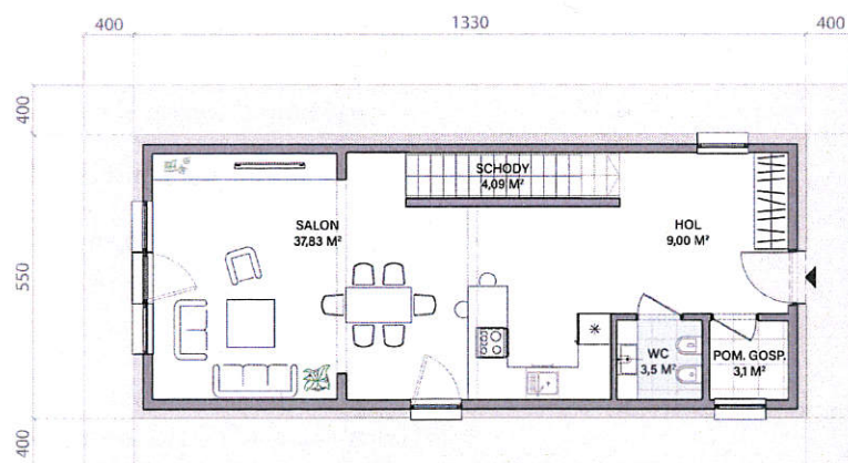
RZUT PARTERU
