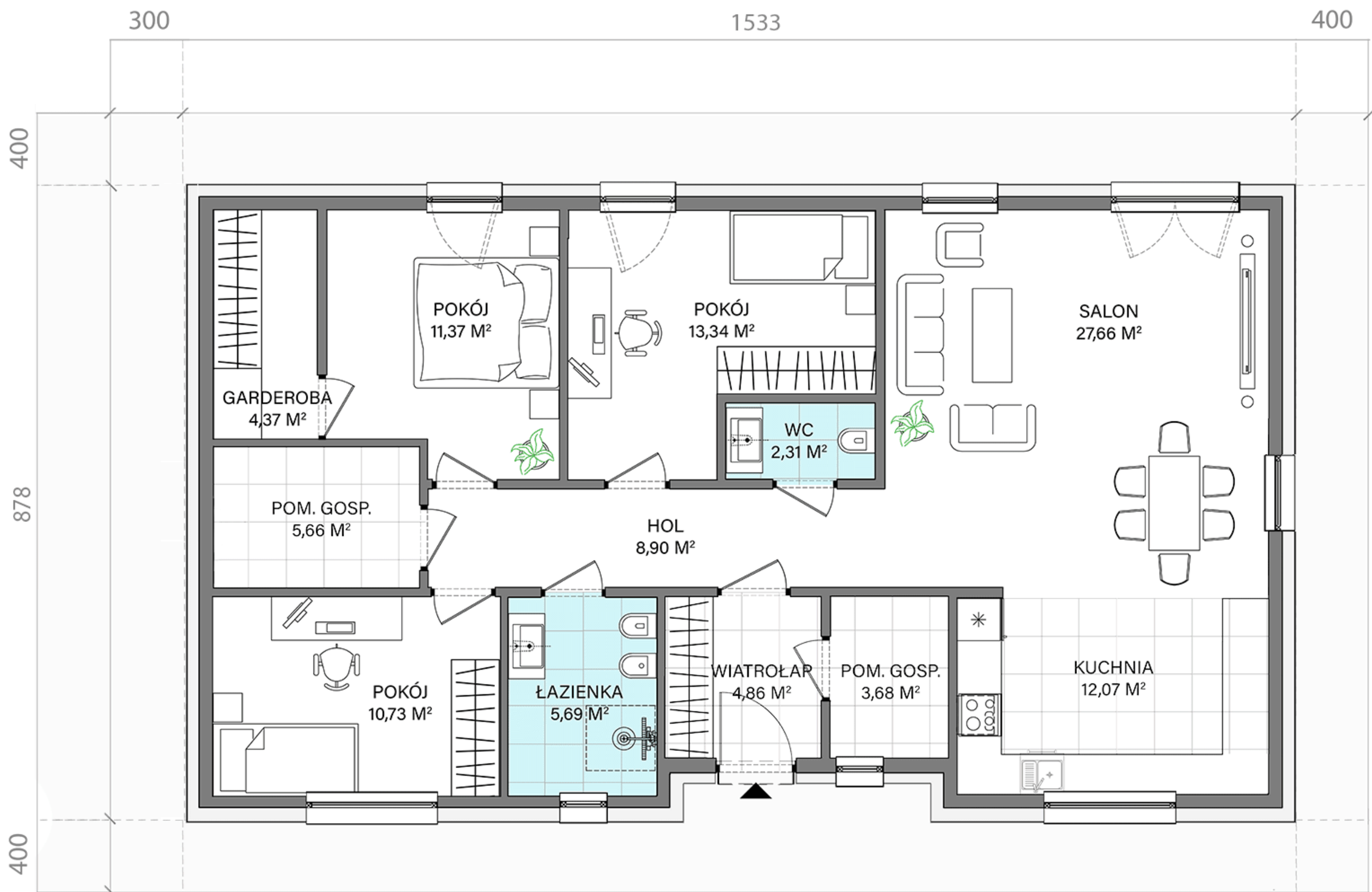
RZUT PARTERU
