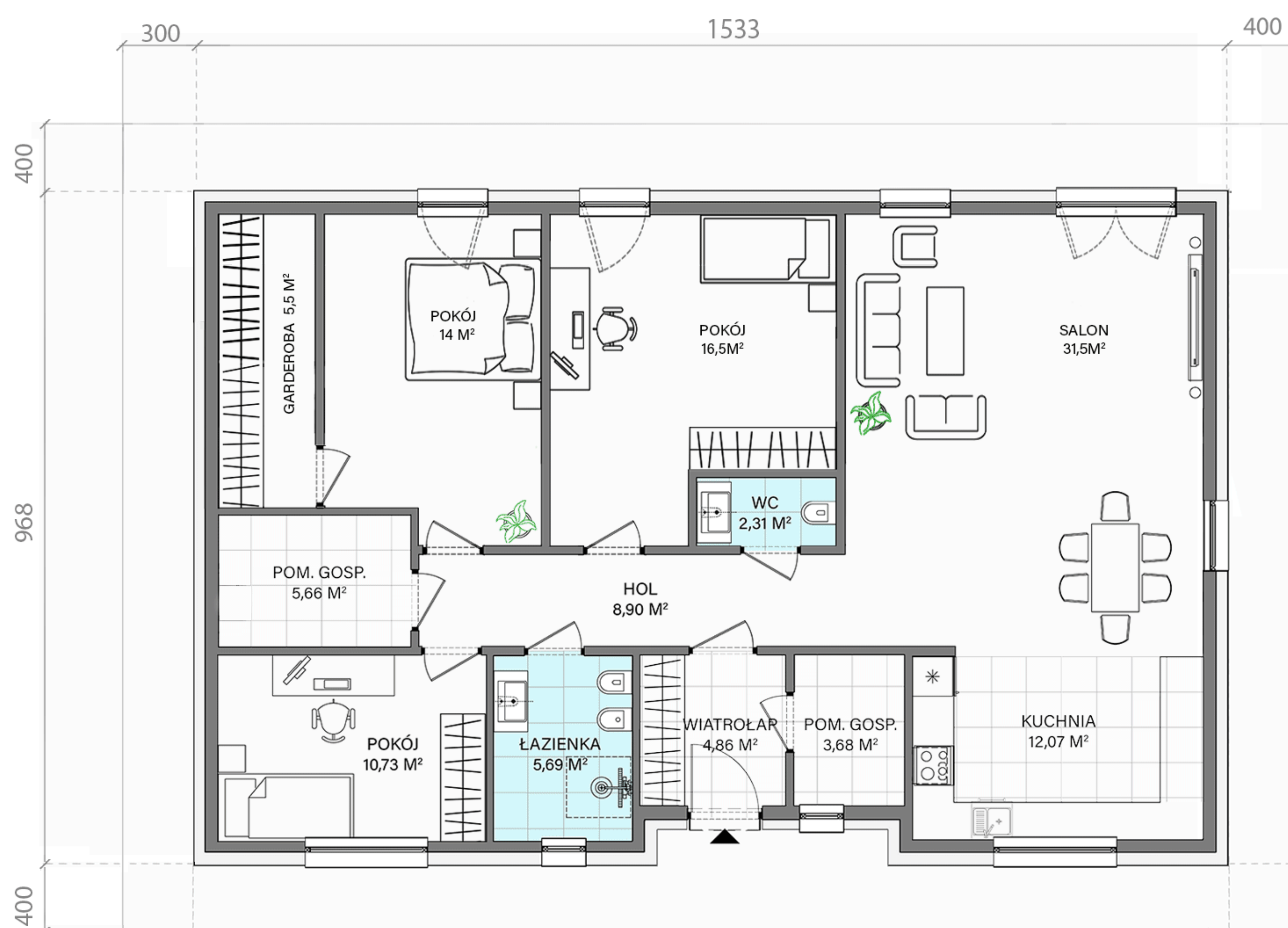
RZUT PARTERU
